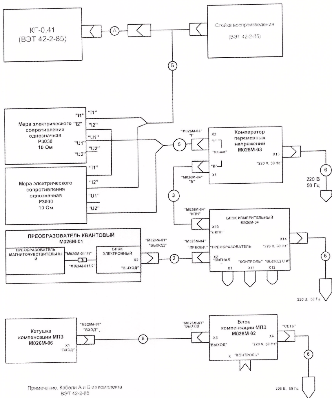
Рисунок 2 - Схема соединений при проверке БИ M026M-04 в диапазоне частот 0,1 – 5 Гц
