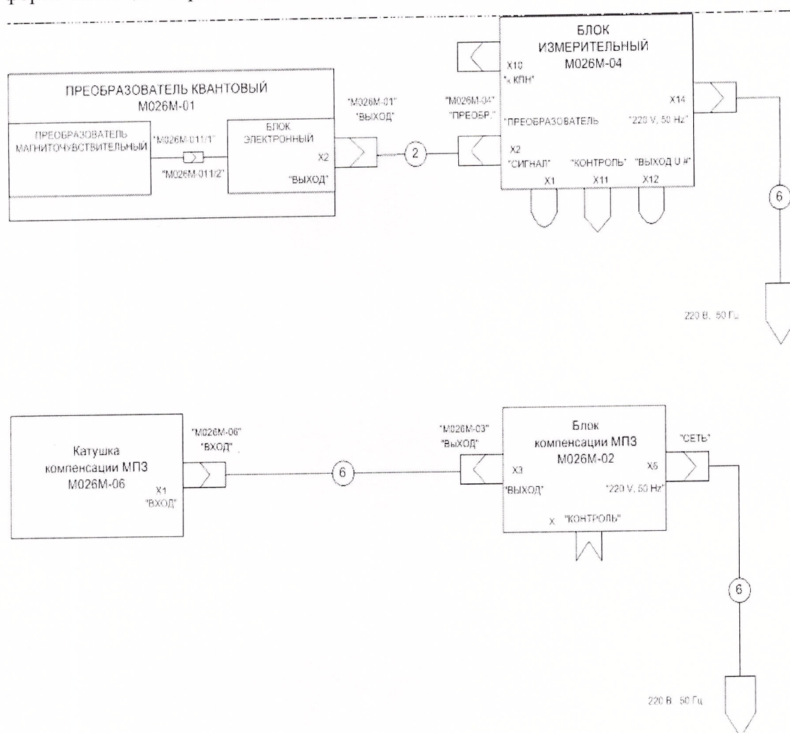
Рисунок 1 - Схема соединений при поверке аппаратуры М026М в постоянном поле
