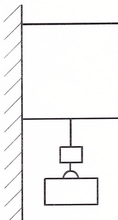
Рисунок 1 - Положение преобразователя при проведении проверок по п. 7.2.2 методики
