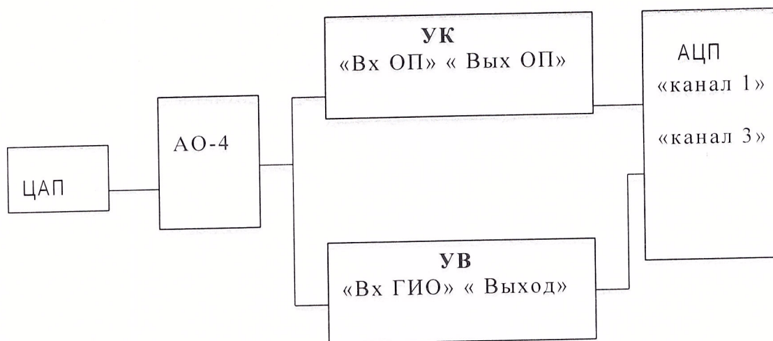
Рис. 6.1 Блок-схема для определения идентичности и линейности приемно-измерительных трактов
