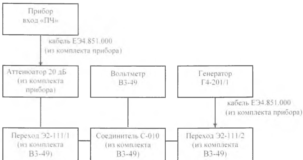
Рисунок 34 - Структурная схема соединения приборов при измерениях параметров АЧХ
