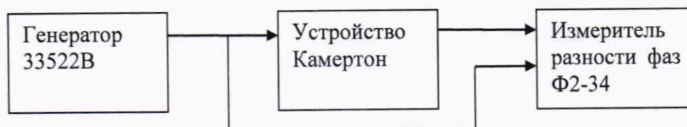
Рисунок 11 Проверка диапазона и абсолютной погрешности воспроизведения добавляемого фазового сдвига между входными и воспроизводимыми выходными синусоидальными сигналами.
