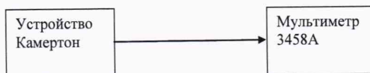
Рисунок 7. Проверка динамического диапазона и относительной погрешности воспроизведения напряжений выходных сигналов в диапазоне выходных напряжений от 50 \cdot 10^3 до 1,5 \cdot 10^6 мкВ.
