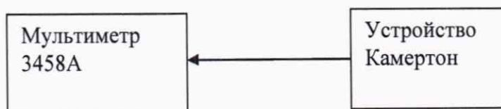
Рисунок 4. Проверка неравномерности АЧХ выходных каналов в диапазоне частот от 0,02 до 20 кГц.
