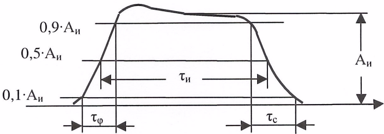
Рисунок 8 – Форма радиоимпульса на экране осциллографа в поддиапазоне частот от 100 до 639 МГц
