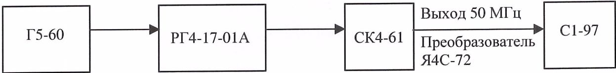
Рисунок 7 – Схема подключения приборов для определения длительностей фронта и среза выходных радиоимпульсов в поддиапазоне частот от 100 до 639 МГц
