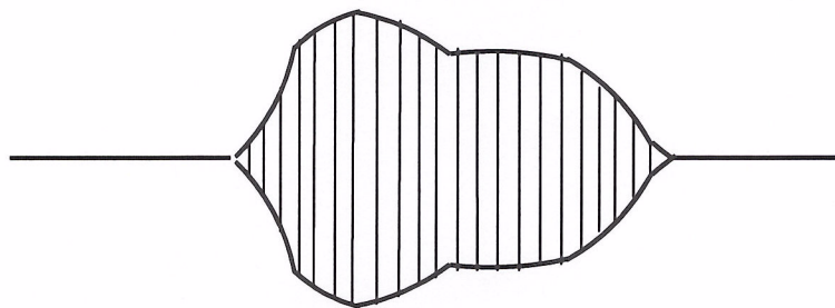
Рисунок 6 – Форма радиоимпульса на экране осциллографа в поддиапазоне частот от 50 до 100 МГц
