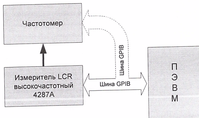
Рисунок 8.1 Схема определения погрешности воспроизведения частоты измерительного сигнала
