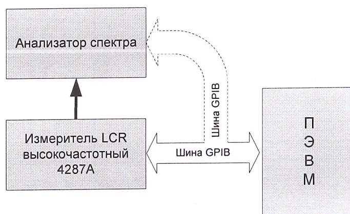
Рисунок 8.2 Определение погрешности воспроизведения мощности выходного измерительного сигнала с использованием анализатора спектра
