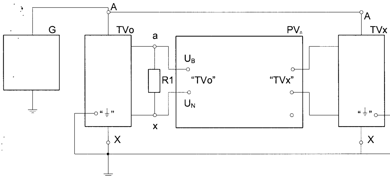
Рисунок 1. Схема поверки методом сличения. G – источник высокого напряжения; TVo - эталонный трансформатор; R1 - нагрузочное устройство; PV Δ - прибор сравнения; TV x – ПВЕ.
