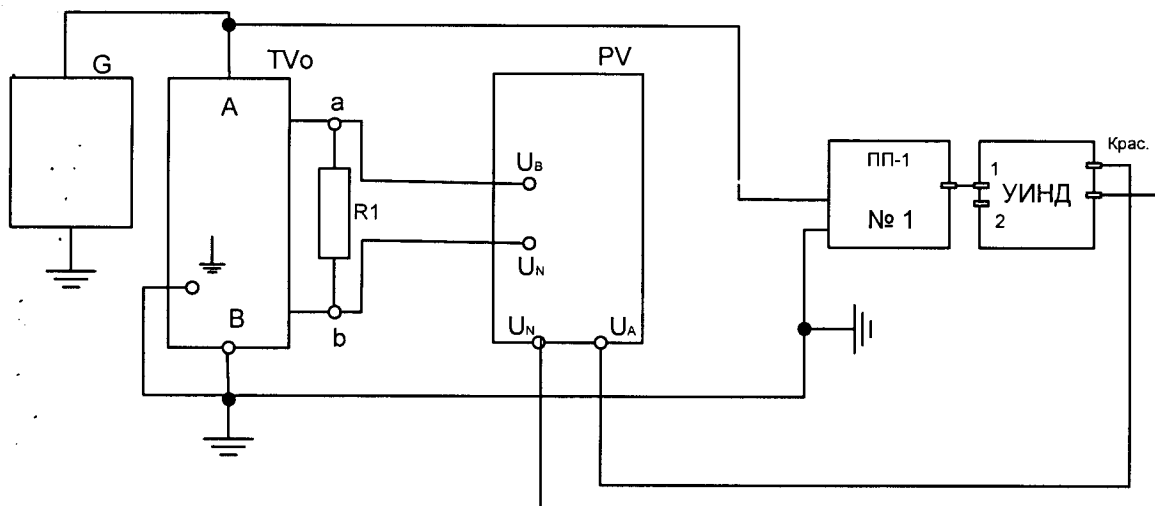
Рисунок 2. Схема поверки первого входа ПВЕ методом сличения. G – источник высокого напряжения; TV 0 - эталонный трансформатор; R1 - нагрузочное устройство; PV - прибор сравнения «Энергомонитор 3.3Т1»; ПП-1 - высоковольтный первичный преобразователь из комплекта ПВЕ; УИНД – усилитель из комплекта ПВЕ.
