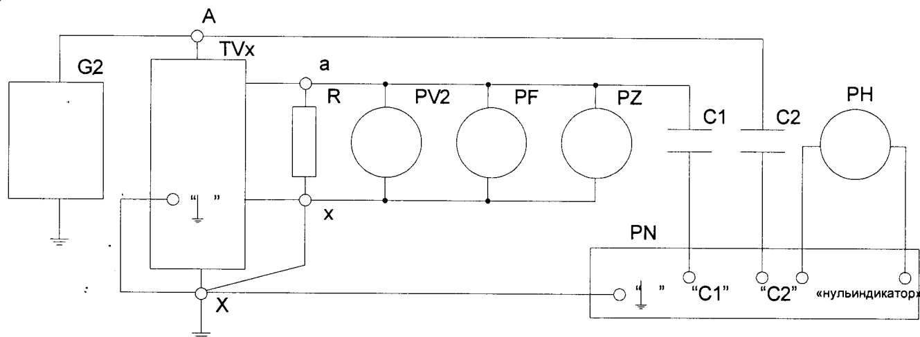
Рисунок 4. Схема поверки методом компарирования токов.
