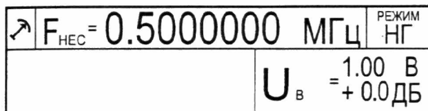
Рис 3. Вид индикатора генератора в режиме немодулированных колебаний.
