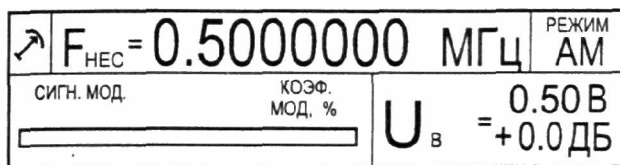
Рис 5. Вид индикатора генератора в режиме амплитудно-модулированных колебаний от внешнего источника.
