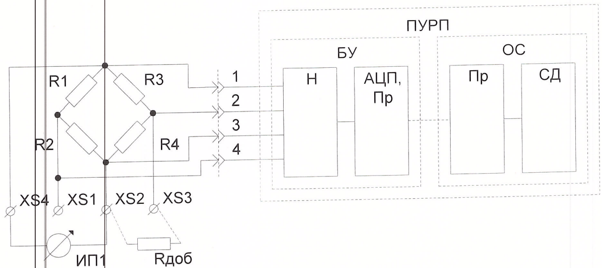
Рис. 1 Схема подключения проверочного оборудования к ИК ПУРП
