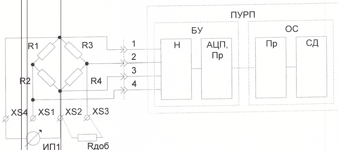
Рис. 1 Схема подключения проверочного оборудования к ИК ПУРП
