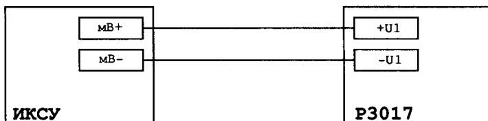
Рисунок 4.5 – Установка для поверки ИКСУ-260 в режиме измерения напряжения
