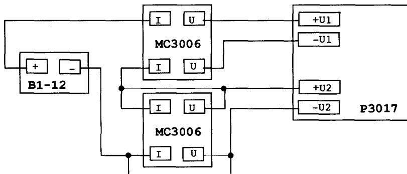
Рисунок 4.6 – Установка для поверки ИКСУ-260 в режиме измерения сопротивления постоянному току
