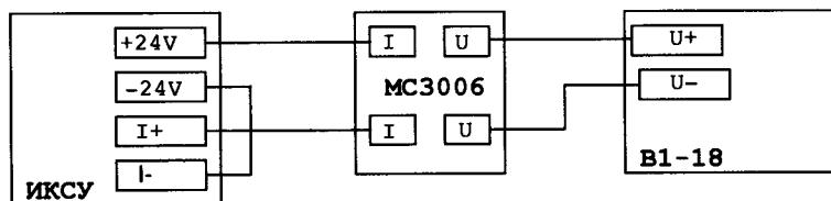
Рисунок 4.4 – Установка для проверки ИКСУ-260 в режиме воспроизведения силы постоянного тока
