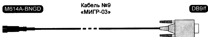
Рисунок А.9. Соединительный кабель №9 для связи ИКСУ с ПК при работе в режиме поверки ПД
