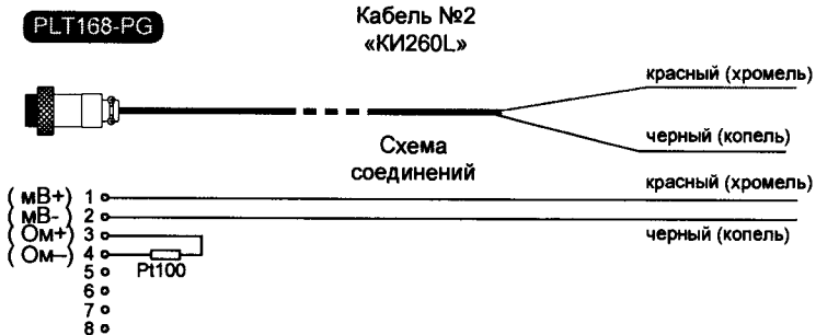
Рисунок А.2. Соединительный кабель №2 для подключения к ИКСУ ТП типа ТХК при работе в режиме измерения температуры, а также для связи с устройствами в режиме воспроизведения сигналов от указанного типа ТП
