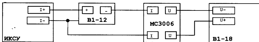
Рисунок 4.8 –Установка для поверки ИКСУ-260 в режиме измерения силы постоянного тока
