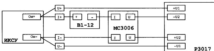
Рисунок 4.3 – Установка для поверки ИКСУ-260 в режиме воспроизведения сопротивления
