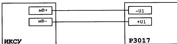
Рисунок 4.1 – Установка для проверки ИКСУ-260 в режиме воспроизведения напряжения (минус10 мВ)
