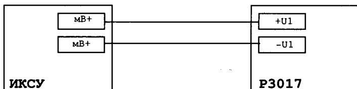
Рисунок 4.2 – Установка для поверки ИКСУ-260 в режиме воспроизведения напряжения (0; 0,022; 2; 30; 60; 100 мВ)
