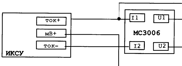
Рисунок 4.7 – Установка для поверки ИКСУ-260 в режиме измерения сопротивления постоянному току
