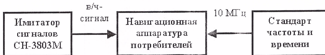
Рис. 8.2.3 Схема рабочего места по пп.8.2.6
