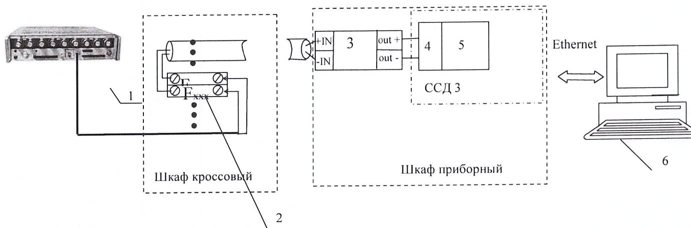
Рис.3. Функциональная схема поверки ИК измерения сопротивления постоянному току в диапазоне от 40 до 130 Ом и от 80 до 200 Ом.
