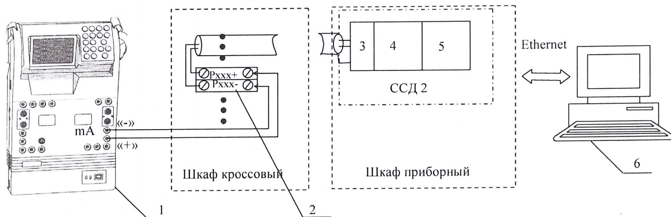
Рис. 1. Функциональная схема поверки ИК измерения напряжения постоянного тока в диапазоне от минус 2 до 55 мВ.
