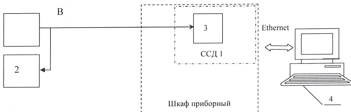
Рис. 5. Функциональная схема поверки ИК измерения напряжения постоянного тока в диапазоне от минус 50 до 50 мВ.
