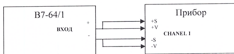
Рис.1. Структурная схема соединения приборов.
