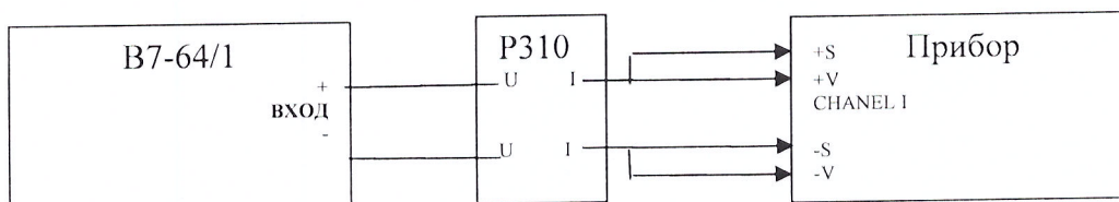
Рис.2. Структурная схема соединения приборов.
