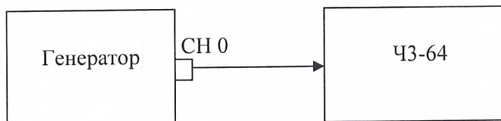
Рисунок 4 - Структурная схема соединения приборов при определении верхних пределов воспроизводимой частоты и погрешности установки частоты
