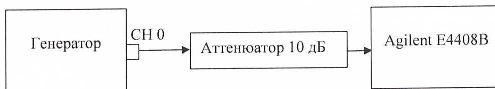
Рисунок 7 - Структурная схема соединения приборов при определении относительного уровня гармонических составляющих и спектральной плотности шума.
