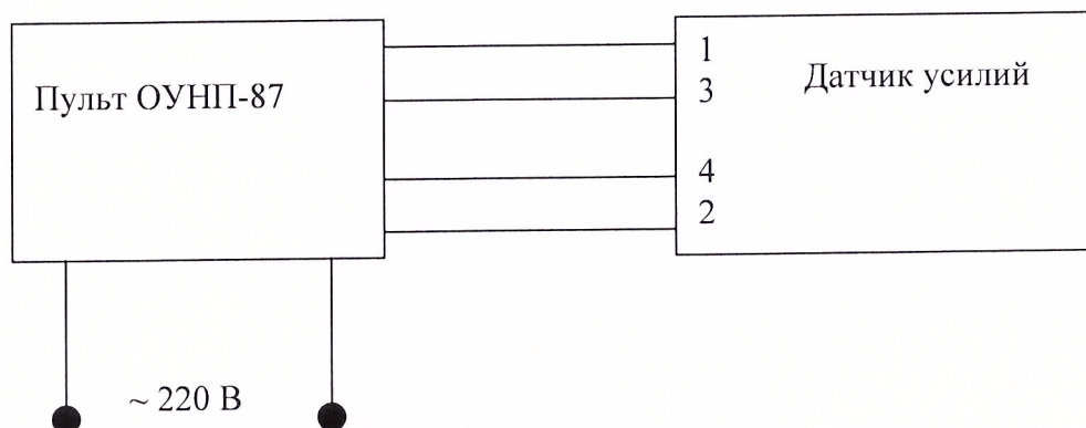
Рисунок 2 - Схема определения градуировочной характеристики датчика
