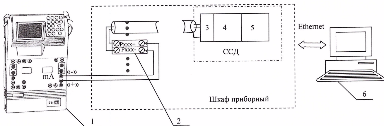
Рис. 1. Функциональная схема поверки ИК измерения напряжения постоянного тока в диапазоне от минус 2 до 55 мВ.
