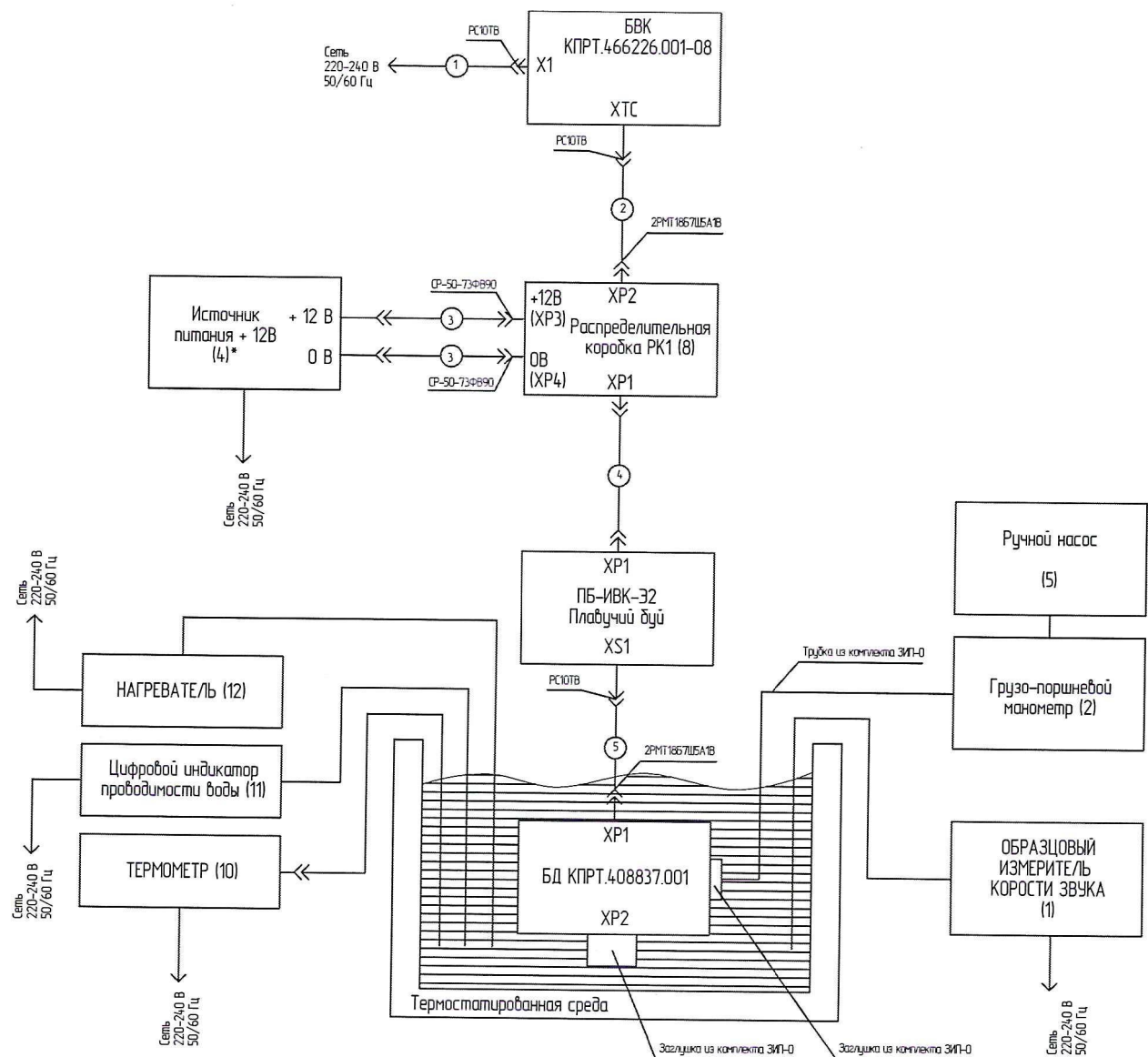
Рис. А.1 – Схема поверки ИВК-Э2.1
