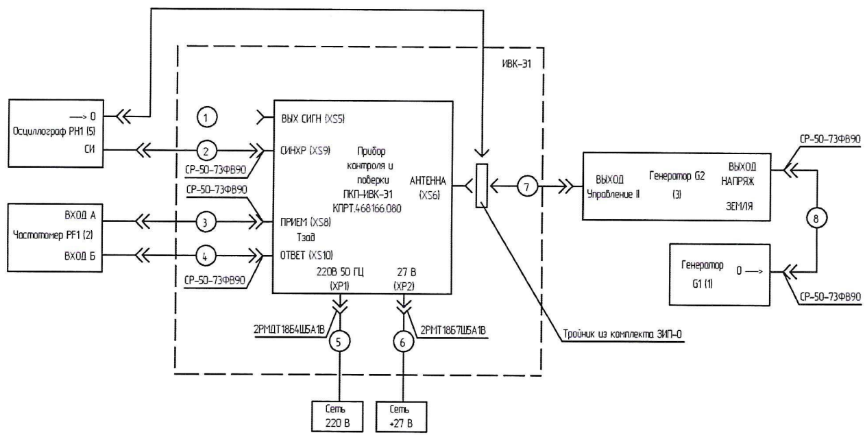
Рис. А.2 – Схема испытаний
