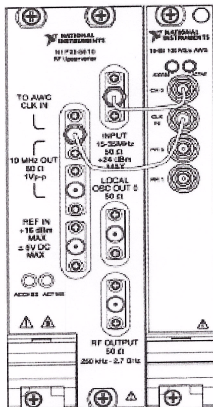
Рисунок 2 - Внешний вид передней панели генератора
