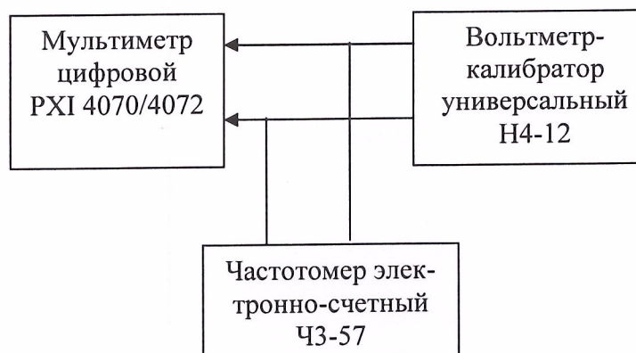
Рисунок 4 - Структурная схема соединения приборов при определении погрешностей измерений частоты
