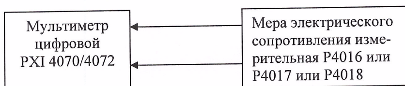
Рисунок 3. Структурная схема соединения приборов при номинальных значениях сопротивления от 1 МОм до 100 МОм.
