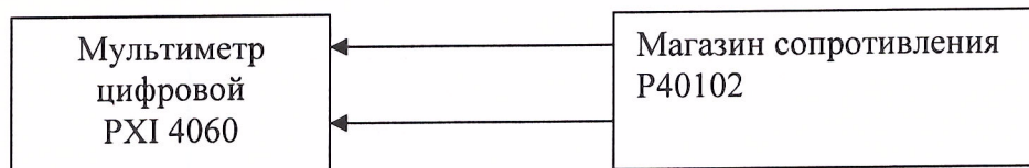
Рисунок 3. Структурная схема соединения приборов при номинальных значениях сопротивления от 150 кОм до 10 МОм.
