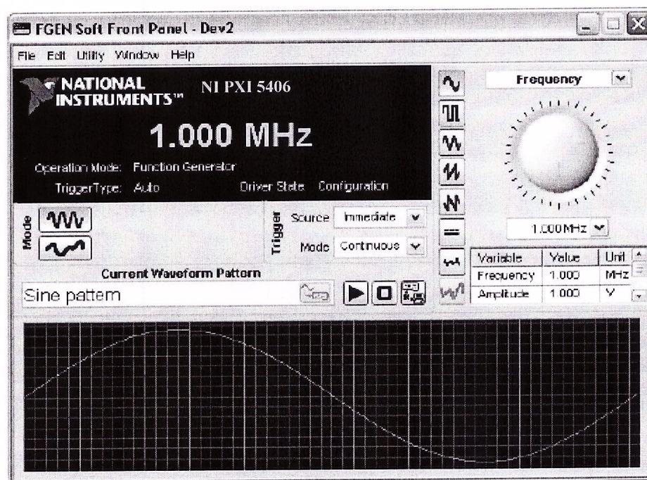
Рисунок 2 - Внешний вид виртуальной панели генератора
