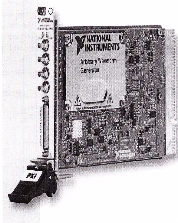
Рисунок 1 - Генератор сигналов произвольной формы PXI-5406
