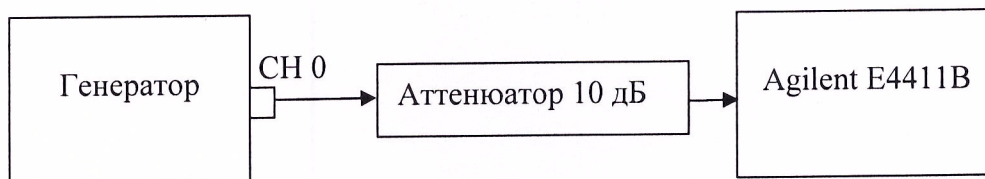
Рисунок 6 – Схема измерений при проверке относительного уровня гармонических составляющих по основному тракту с высоким усилением
