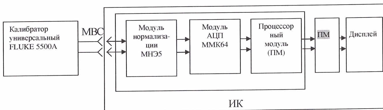
Рисунок 8 – Функциональная схема поверки ИК системы «Ангара-11356»
