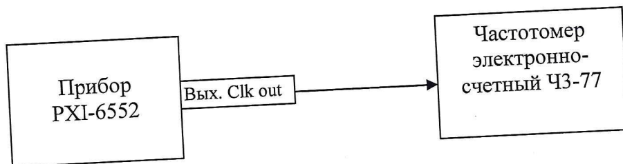
Рисунок 6.2 - Структурная схема соединения приборов
