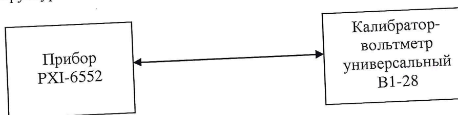
Рисунок 6.1 - Структурная схема соединения приборов
