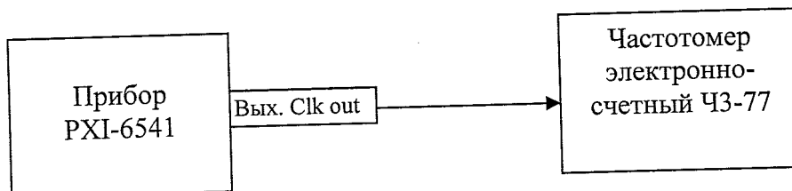
Рисунок 5.2 - Структурная схема соединения приборов
