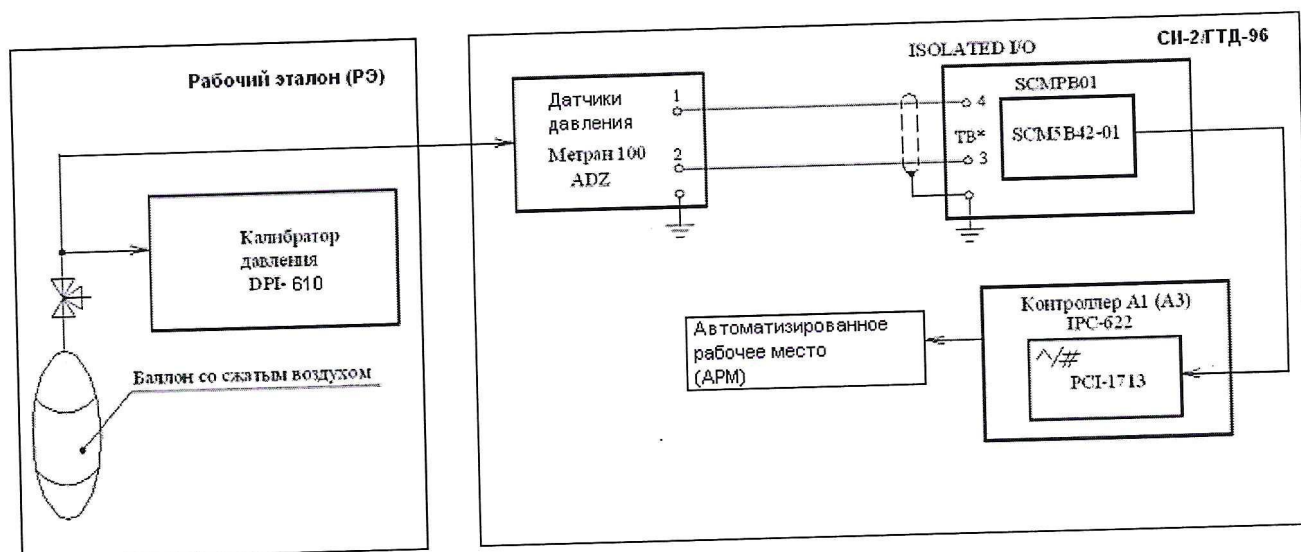
Рисунок 1 – Схема комплектной поверки ИК давления рабочим эталоном DPI-610
