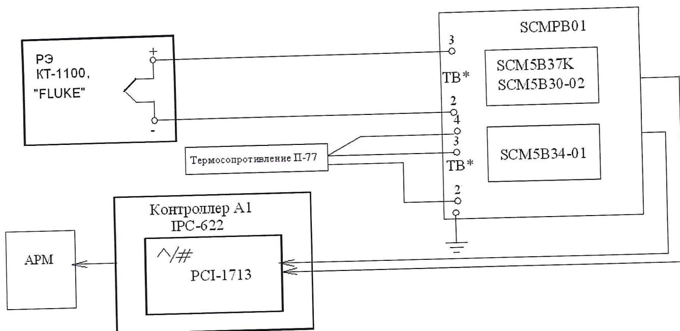
Рисунок 6 – Схема комплектной поверки ИК температуры с термоэлектрическими преобразователями ХА, ХК рабочими эталонами «FLUKE», «КТ-1100»
