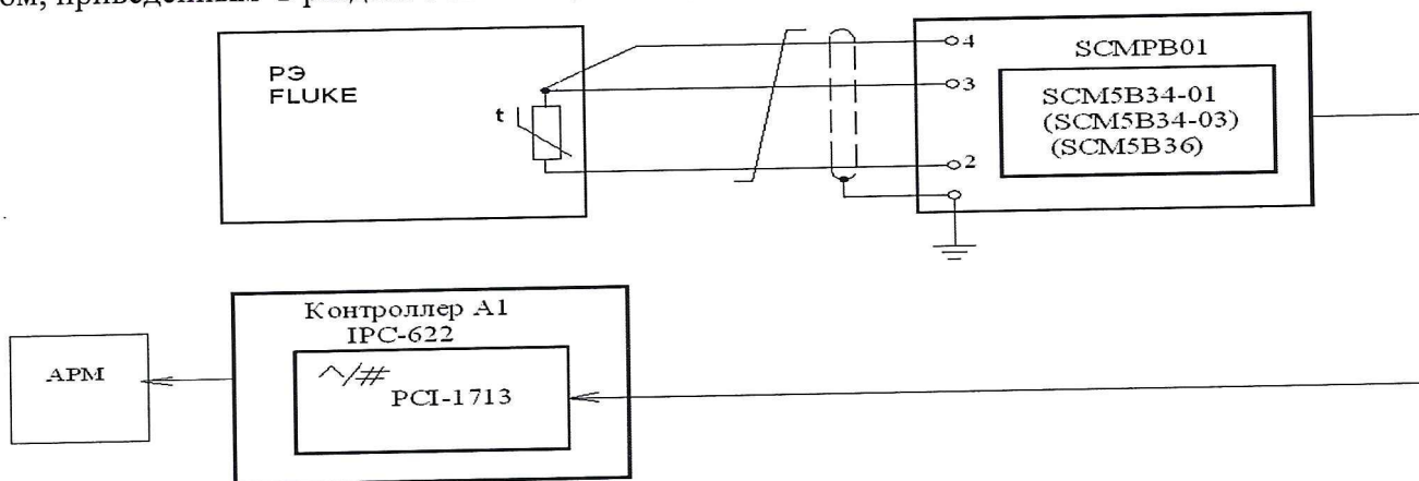
Рисунок 4 – Схема комплектной поверки ИК температуры с термометрами сопротивления
