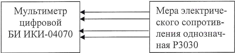
Рисунок 6.2. Структурная схема соединения приборов при номинальных значениях сопротивления от 100 Ом до 100 кОм
