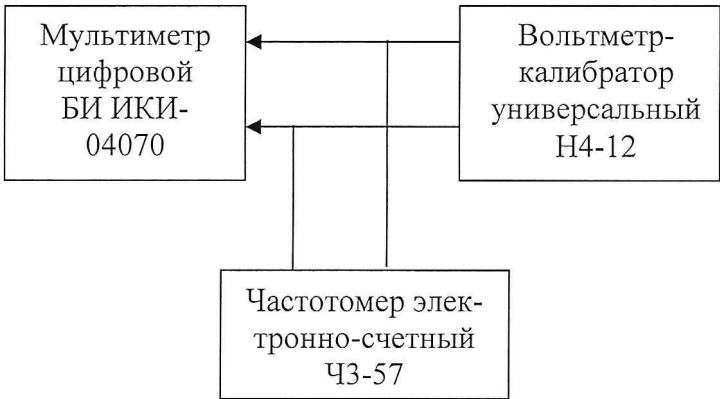
Рисунок 6.4 - Структурная схема соединения приборов при определении погрешностей измерений частоты
