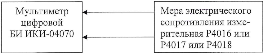
Рисунок 6.3. Структурная схема соединения приборов при номинальных значениях сопротивления от 1 МОм до 100 МОм.
