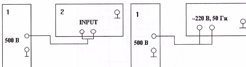
1 – мегаомметр; 2 – проверяемый прибор
