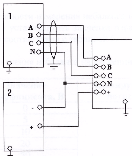
1 – Многофункциональный калибратор переменного напряжения и тока «Ресурс-К2»; 2 – источник питания постоянного тока Б5-49; 3 – проверяемый прибор
