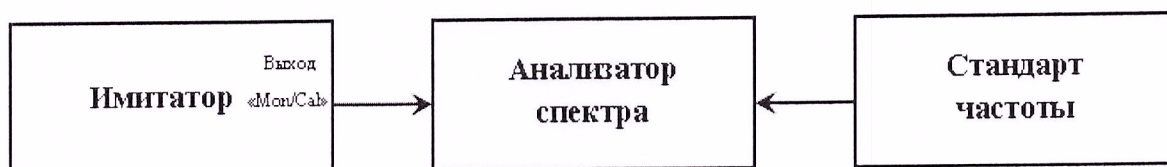
Рисунок 1 – Схема измерений для определения номинальных значений несущих частот выходных сигналов
