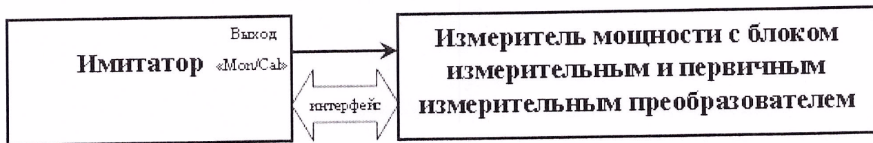
Рисунок 3 – Схема измерений для определения максимального уровня мощности выходных сигналов
