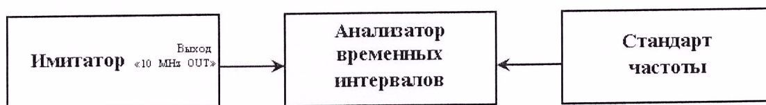
Рисунок 2 – Схема измерений для определения относительной вариации частоты внутреннего опорного генератора
