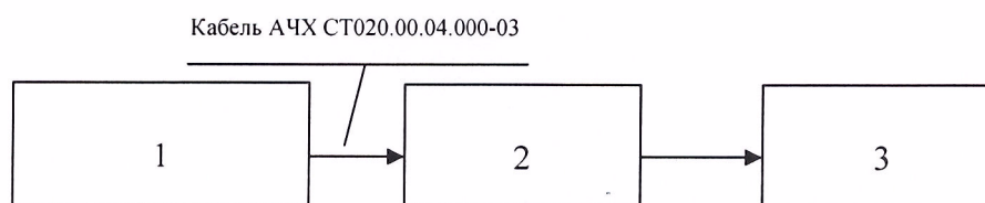
Рисунок 2 – Функциональная схема ИК температуры
