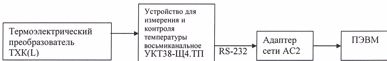
Рисунок 2 – Функциональная схема ИК температуры
