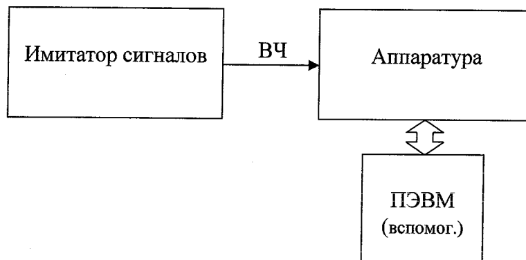
Рисунок 1 - Схема измерений для поверки аппаратуры
