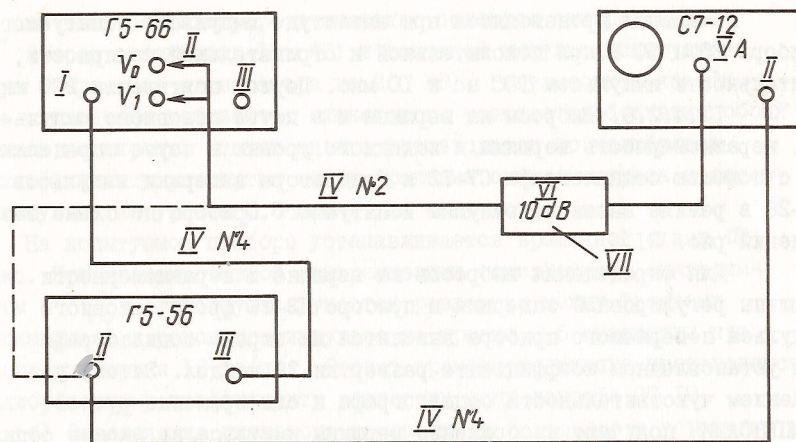
Рис.35. Схема соединения приборов для измерения параметров синхроимпульсов: I - ВНЕШ.ЗАПУСК; II - СИНХР.; III - выход; IV - кабель ИВ4; V - вход; VI - аттенюатор; VII - из комплекта ЗИП осциллографа С7-12
