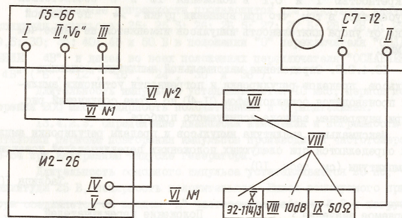
Рис.31. Схема соединения приборов при работе с осциллографом С7-12 и генератором задержки измерителя временных интервалов И2-26:
