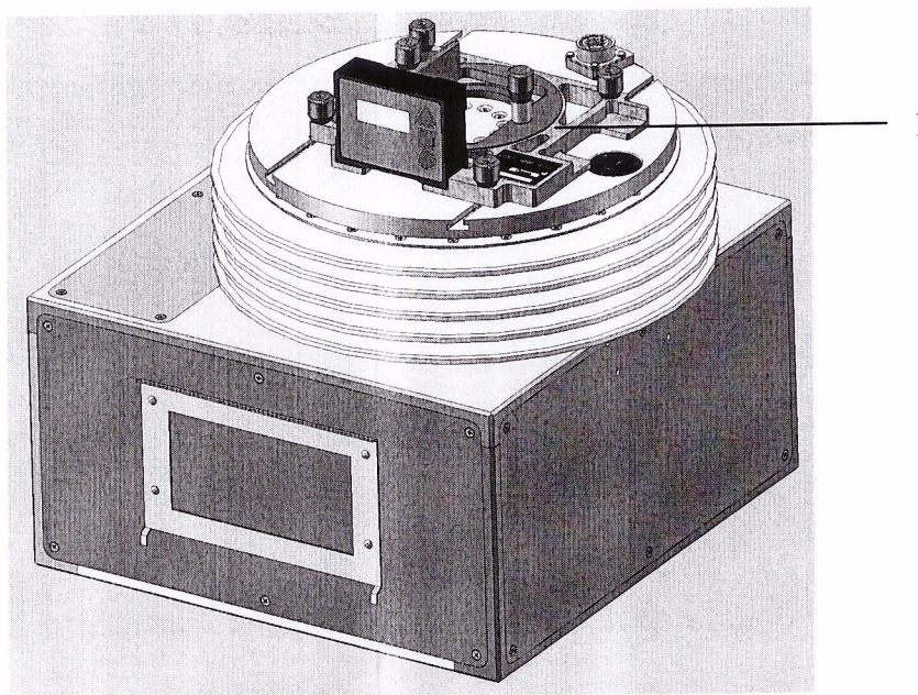
1 – Опора СПАН.301322.002
