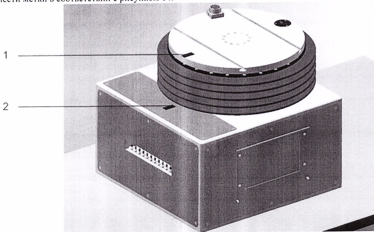
Рисунок 14 – Пример расположения меток на краю платформы приборной и верхней поверхности поворотного блока
