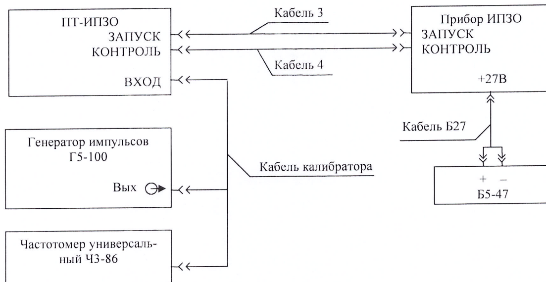
Рисунок 10 - Определение погрешности измерений временных характеристик видеосигналов
