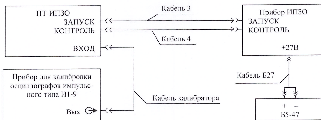
Рисунок 8 - Определение относительной погрешности измерений амплитуды импульсов
