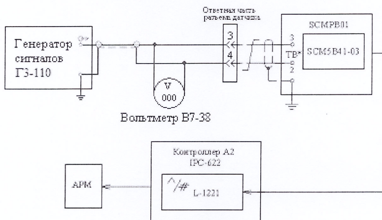
Рисунок 24 – Схема поверки ИК параметров вибрации без ПИП рабочими эталонами ГЗ-110, В7-38
