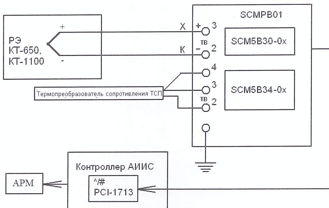
Рисунок 16 – Схема комплектной поверки ИК температуры с термоэлектрическими преобразователями ТХК(L) и платой АЦП PCI-1713 рабочими эталонами КТ-650, КТ-1100
