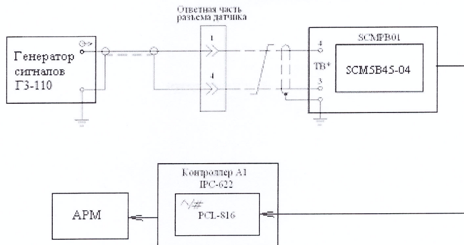
Рисунок 20 – Схема комплектной поверки ИК частоты электрических сигналов, соответствующей частоте вращения роторов рабочим эталоном ГЗ-110
