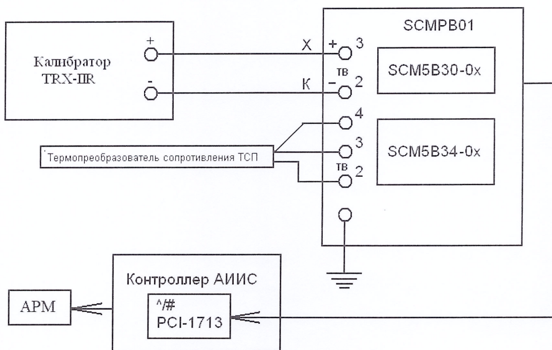
Рисунок 18 – Схема поверки ИК температуры с платой АЦП PCI-1713 без термоэлектрического преобразователя ТХК(L) рабочим эталоном TRX-IIR
