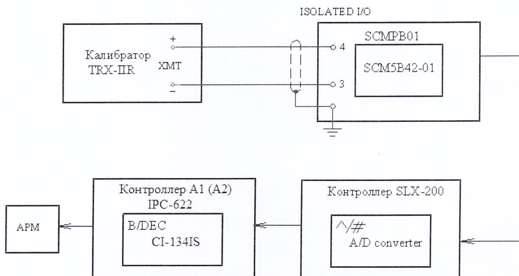
Рисунок 7 – Схема поверки ИК давления с контроллером SLX-200 без датчика давления рабочим эталоном TRX-IIR
