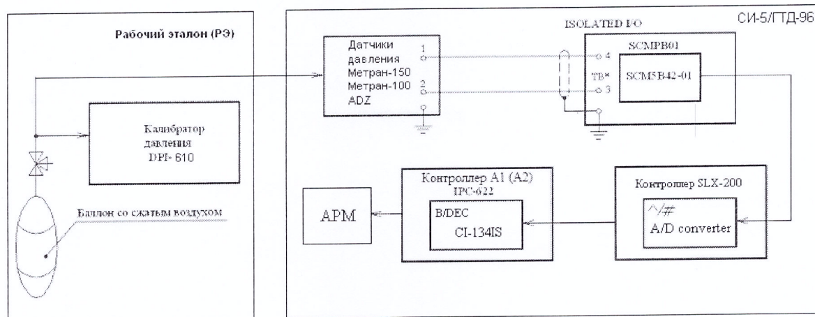
Рисунок 5 – Схема комплектной поверки ИК давления с контроллером SLX-200 рабочим эталоном DPI 610
