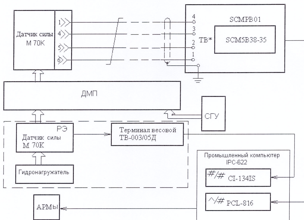
Рисунок 22 – Схема комплектной поверки ИК силы от тяги рабочим эталоном (датчик силы М70К) и СГУ
