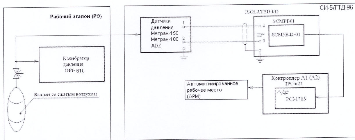
Рисунок 4 – Схема комплектной поверки ИК давления с платой АЦП PCI-1713 рабочим эталоном DPI 610
