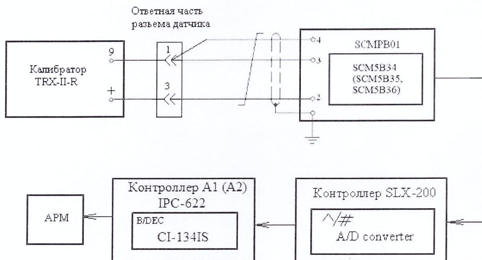
Рисунок 11 – Схема поверки ИК температуры с контроллером SLX-200 без термопреобразователя сопротивления рабочим эталоном TRX-IIR
