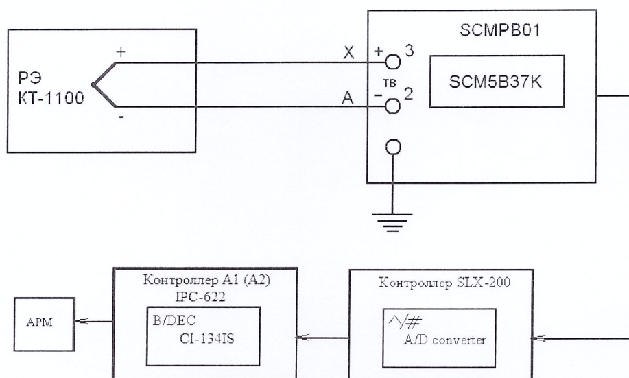
Рисунок 13 – Схема комплектной поверки ИК температуры с термоэлектрическими преобразователями ТХА(К) и контроллером SLX-200 рабочим эталоном КТ-1100
