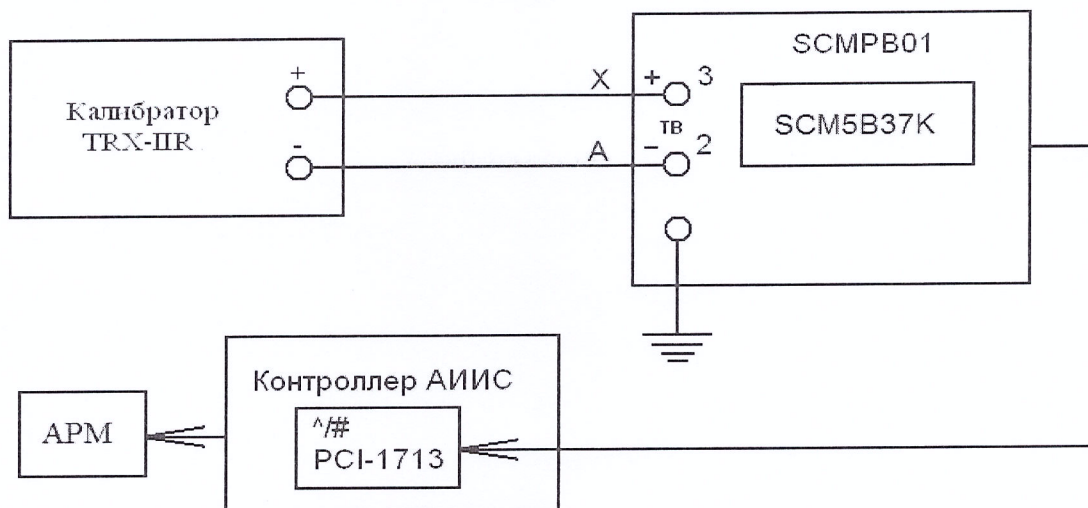
Рисунок 14 – Схема поверки ИК температуры с платой АЦП PCI-1713 без термоэлектрического преобразователя ТХА(К) рабочим эталоном TRX-IIR
