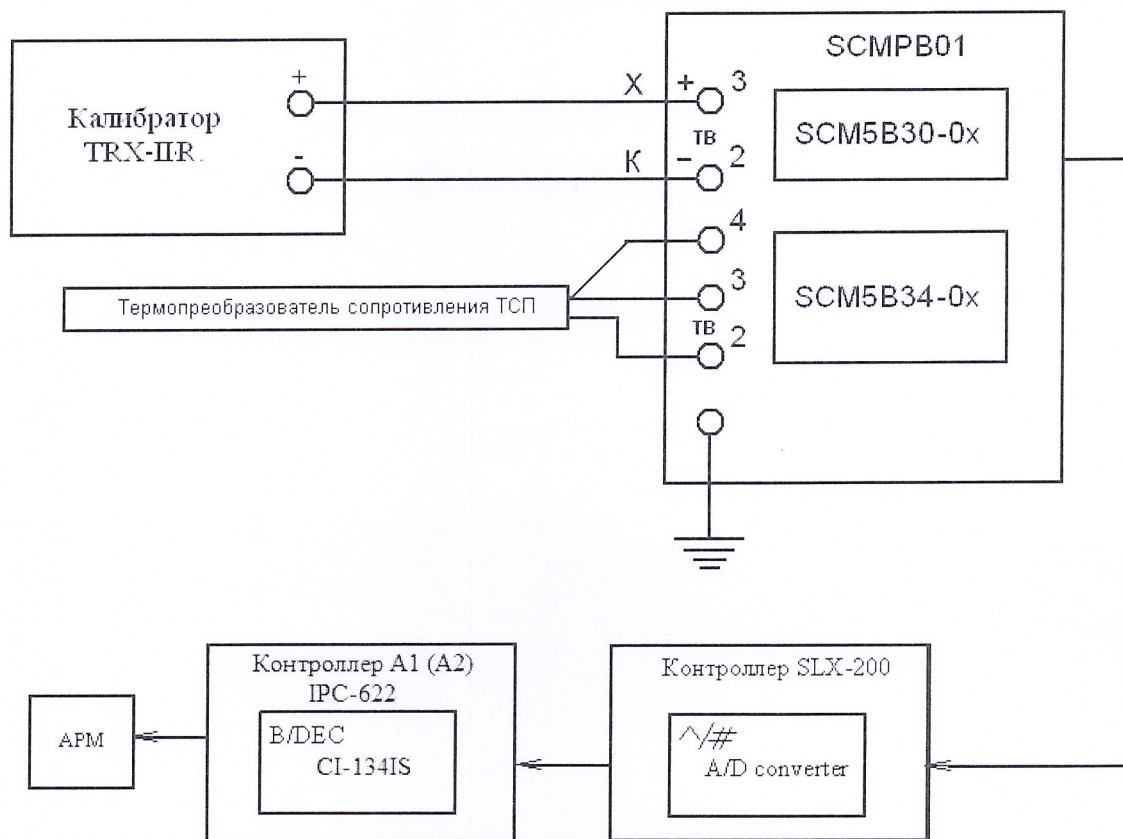
Рисунок 19 – Схема поверки ИК температуры с контроллером SLX-200 без термоэлектрического преобразователя ТХК(L) рабочим эталоном TRX-IIR
