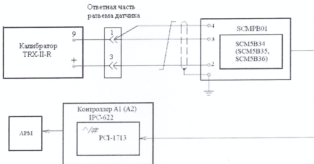
Рисунок 10 – Схема поверки ИК температуры с платой АЦП PCI-1713 без термопреобразователя сопротивления рабочим эталоном TRX-IIR
