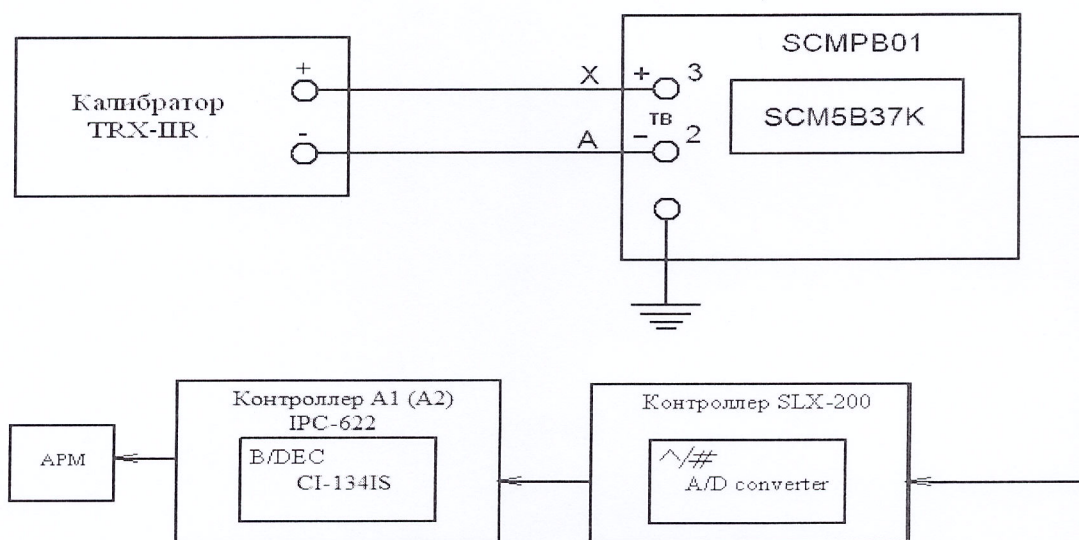
Рисунок 15 – Схема поверки ИК температуры с контроллером SLX-200 без термоэлектрического преобразователя ТХА(К) рабочим эталоном TRX-IIR
