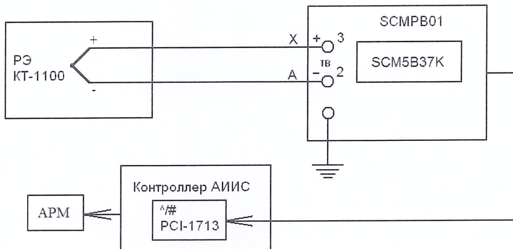
Рисунок 12 – Схема комплектной поверки ИК температуры с термоэлектрическими преобразователями ТХА(К) и платой АЦП PCI-1713 рабочим эталоном КТ-1100
