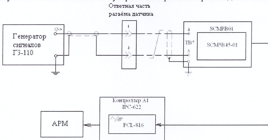
Рисунок 21 – Схема комплектной поверки ИК расхода (прокачки) масла рабочим эталоном ГЗ-110
