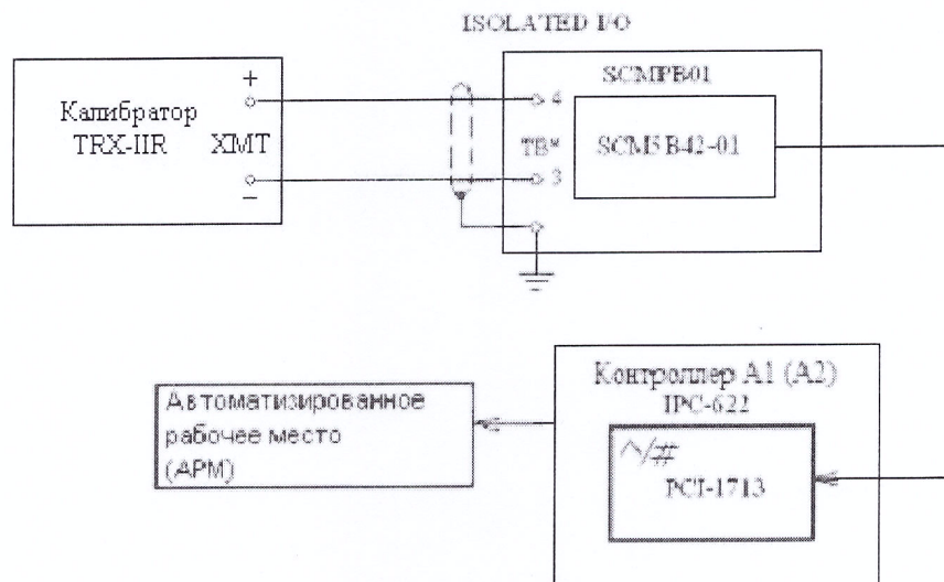
Рисунок 6 – Схема поверки ИК давления с платой АЦП PCI-1713 без датчика давления рабочим эталоном TRX-IIR
