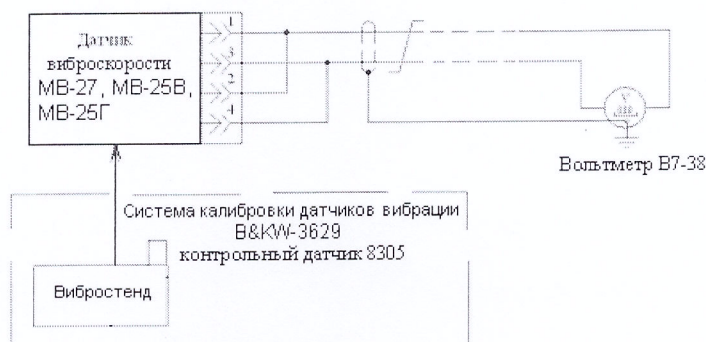
Рисунок 23 – Схема поверки датчиков виброскорости МВ-27, МВ-25В, МВ-25Г рабочими эталонами 8305, В7-38
