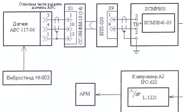
Рисунок 25 – Схема поверки ИК вибрации с датчиками виброускорения ABC-117-06 рабочим эталоном HI-803
