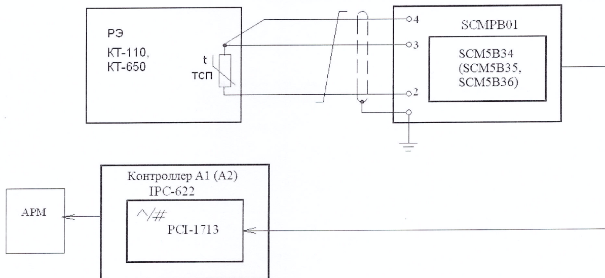
Рисунок 8 – Схема комплектной поверки ИК температуры с термопреобразователями сопротивления и платой АЦП PCI-1713 рабочими эталонами КТ-110, КТ-650
