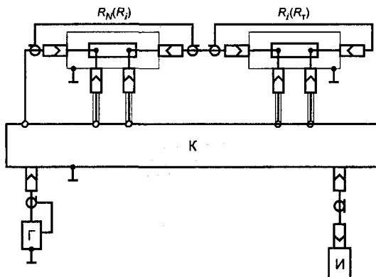
Г — генератор; К — компаратор; И — индикатор равновесия
