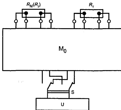
Рисунок Б.1 — Подключение сравниваемых мер при использовании метода замещения
