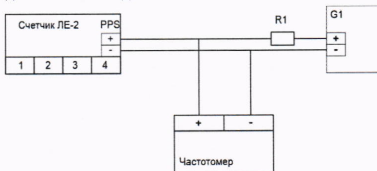
Рисунок 4 - Где G1 - источник постоянного напряжения; R1 - резистор 2 кОм \pm 5\% .
