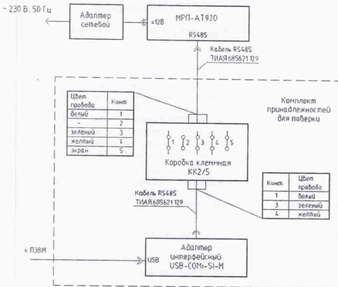
Рисунок 11 – Схема подключения МРП-АТ920, МРП-АТ920В, МРП-АТ920Р к ПЭВМ при помощи комплекта принадлежностей для поверки
