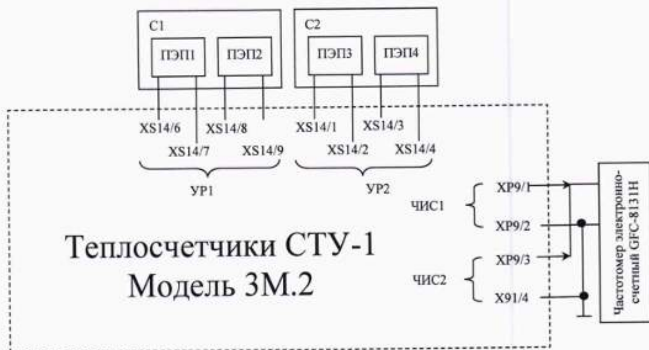
Рисунок 10.3.1 - Схема поверки теплосчетчика СТУ-1 Модель 3М.1 проливным методом
