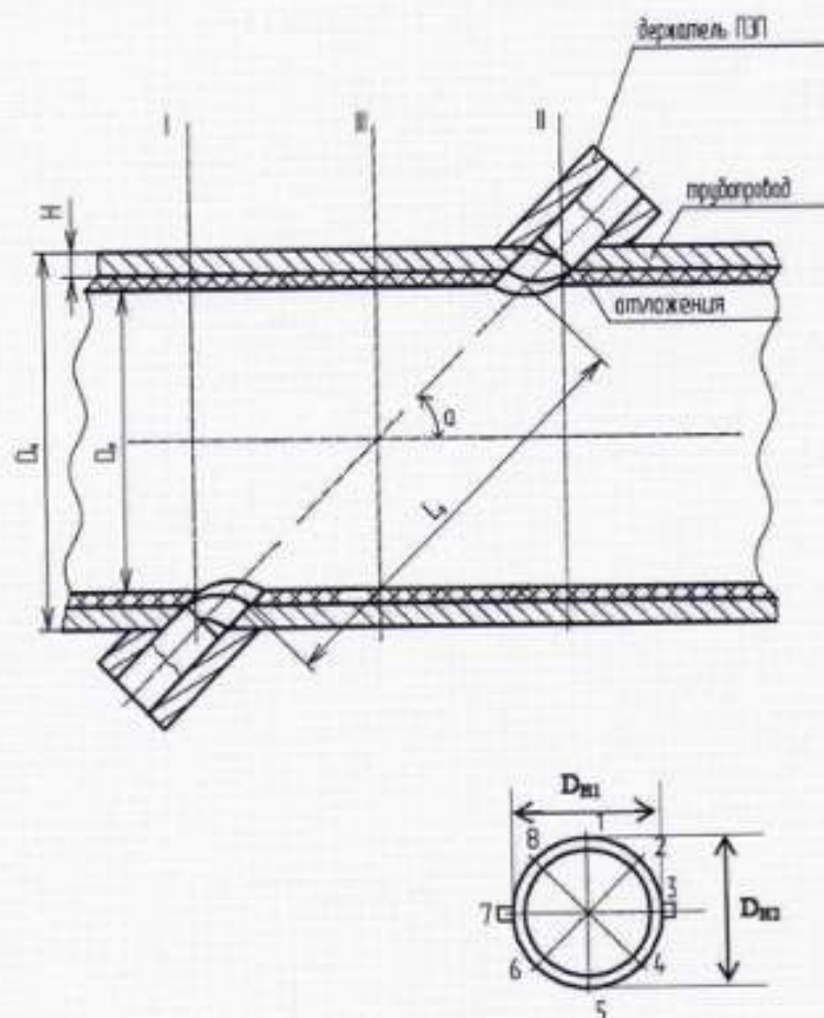
Рисунок 10.2.4 - Эскиз к процедуре измерения длины активной части акустического канала
