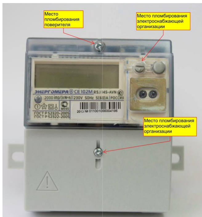
Рисунок 4 - Общий вид счетчика CE102M R5.1
