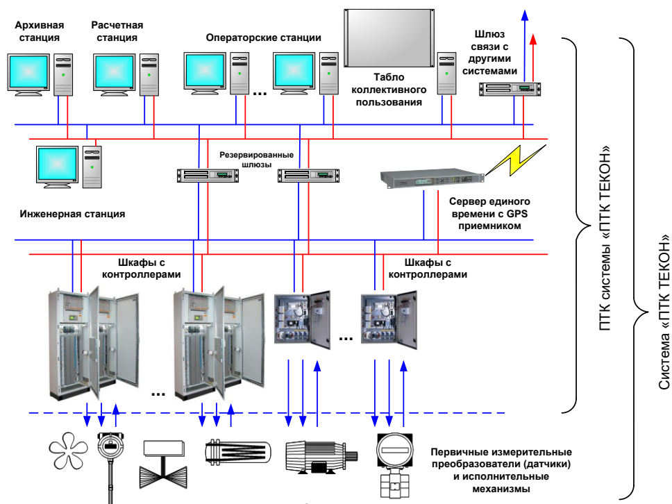
Рисунок 1 — Обобщенная структурная схема систем «ПТК ТЕКОН»
