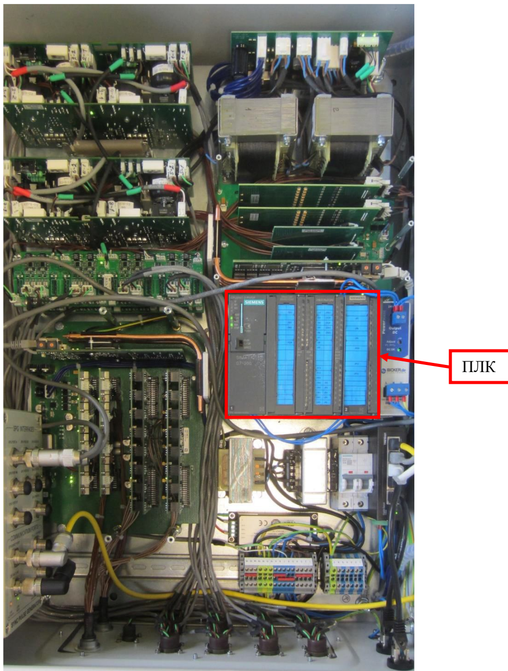
Рисунок 3 – Общий вид блоков электроники и ПЛК внутри шкафа
