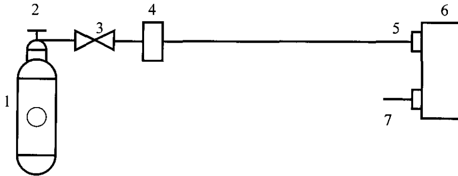
Рис.Д1. Схема проверки основной погрешности газоанализатора.
