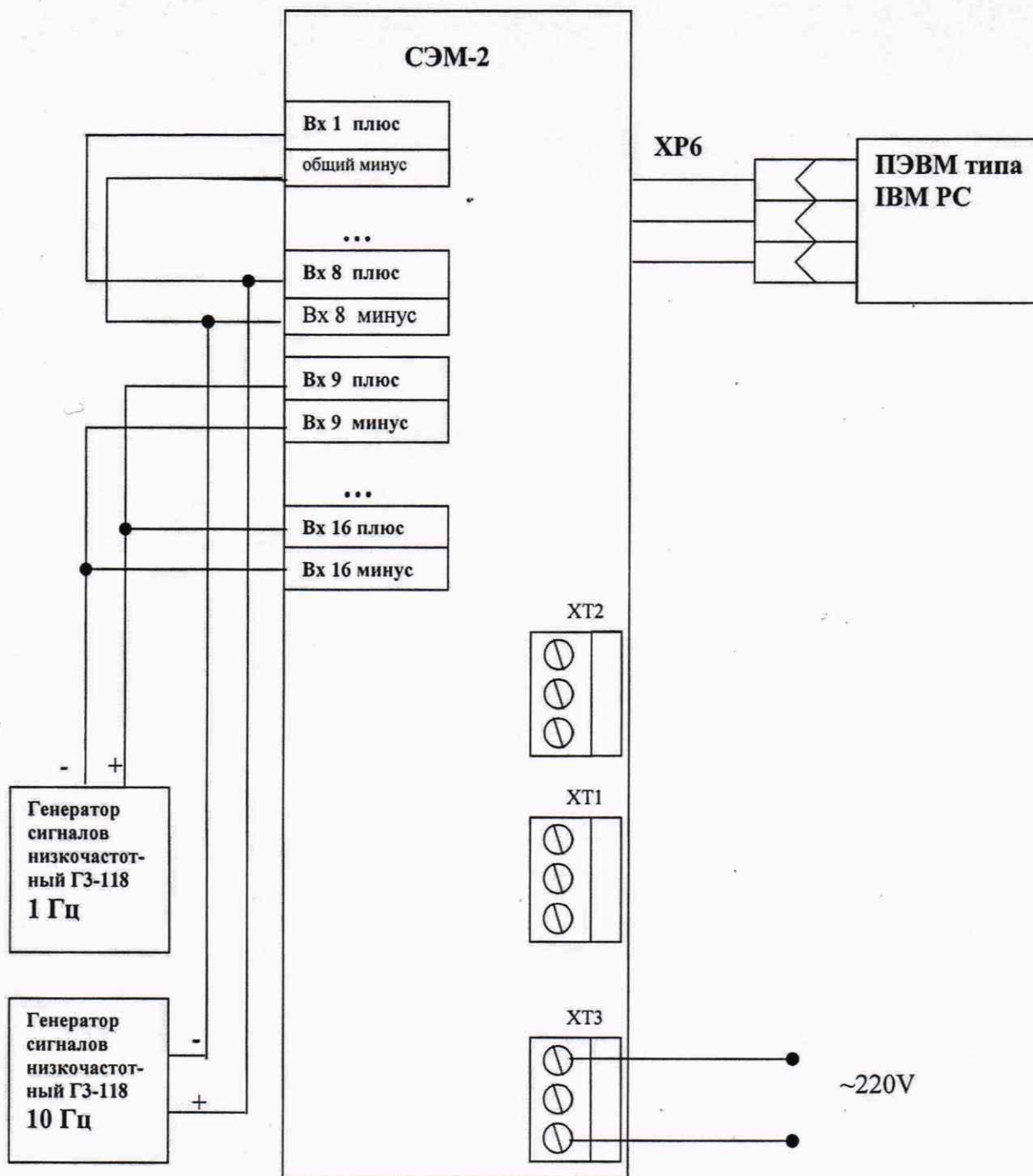
Рисунок Б.1 - Схема коммутации сумматора для первичной поверки после выпуска из производства или после ремонта
