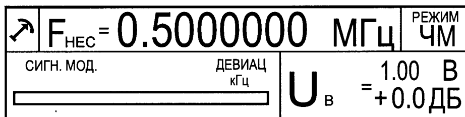
Рис 7. Вид индикатора генератора в режиме частотно-модулированных колебаний от внешнего генератора.
