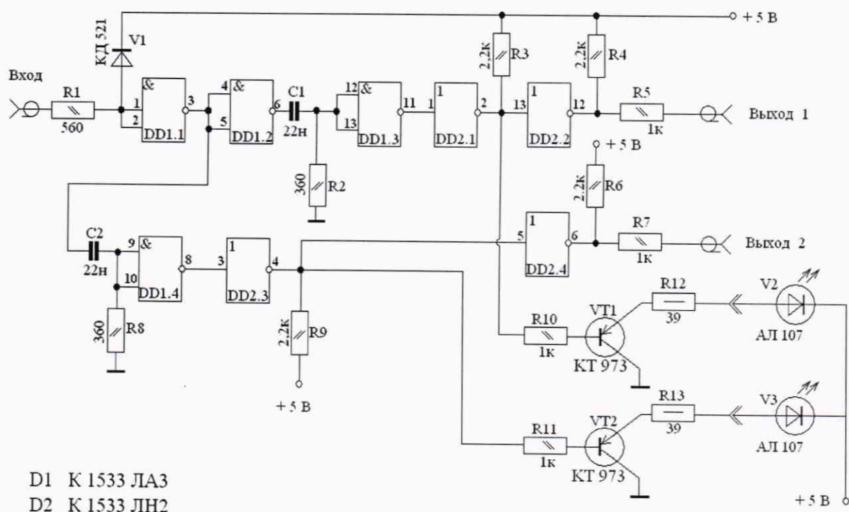
Рисунок 3 - Вспомогательная схема
