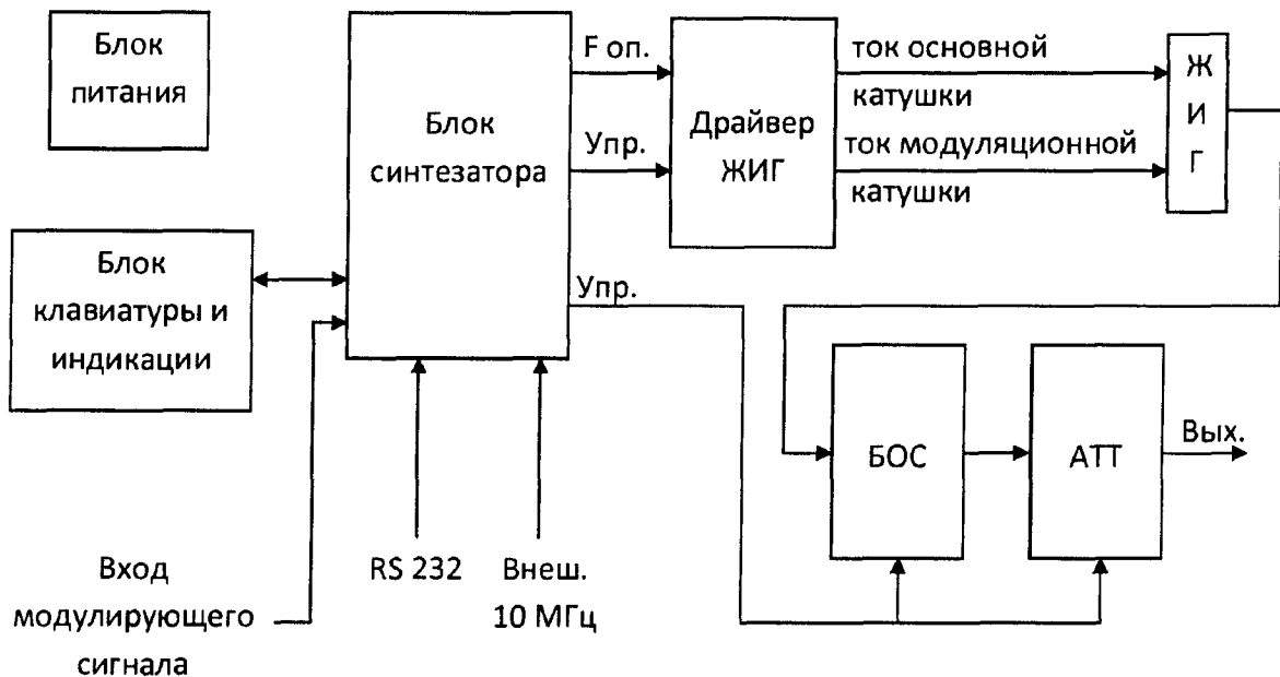
Рис 4.1. Структурная схема генератора
