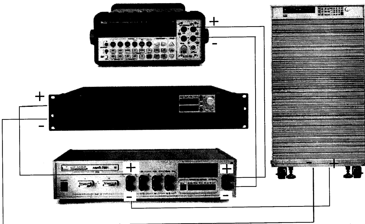
Рисунок 1 Структурная схема соединения приборов для определения абсолютной погрешности установки постоянного тока и измерения силы постоянного тока
