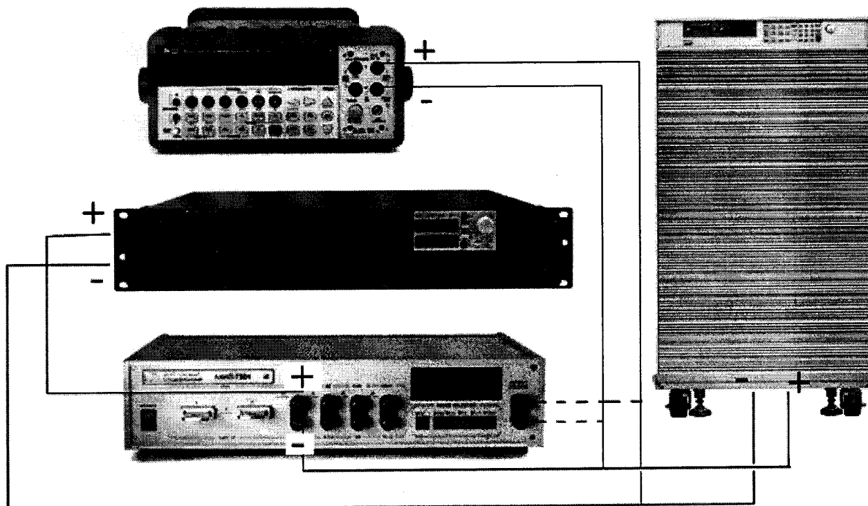
Рисунок 3 Структурная схема соединения приборов для определения абсолютной погрешности установки и измерения мощности и установки сопротивления
