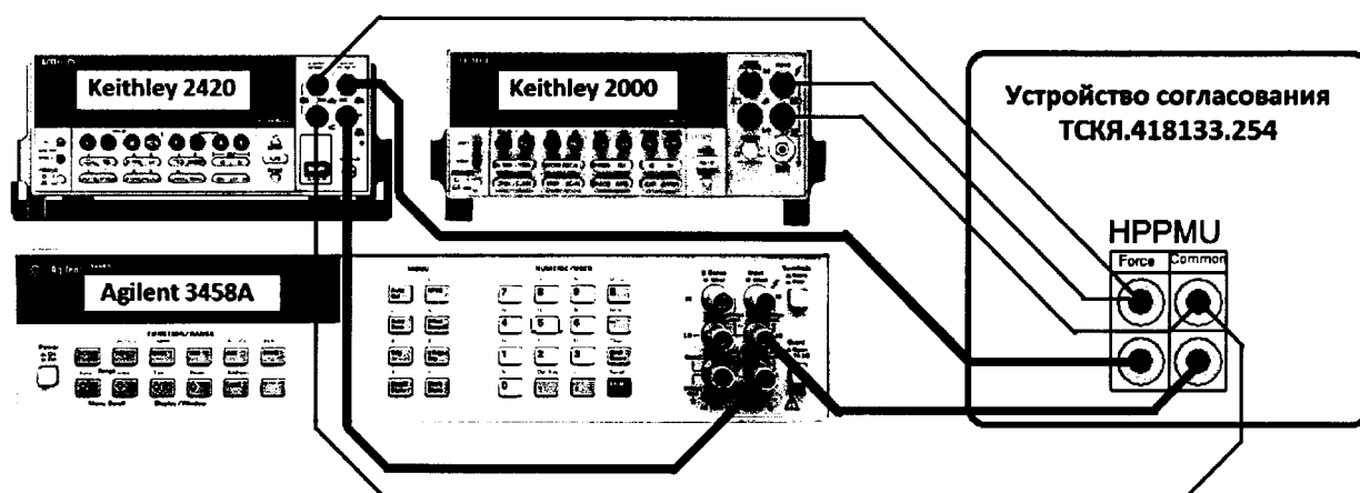
Рисунок 22 – Схема определения погрешности воспроизведения (измерения) напряжения и измерения (воспроизведения) силы тока HPPMU при подключении через разъем UTILITY pogo block
