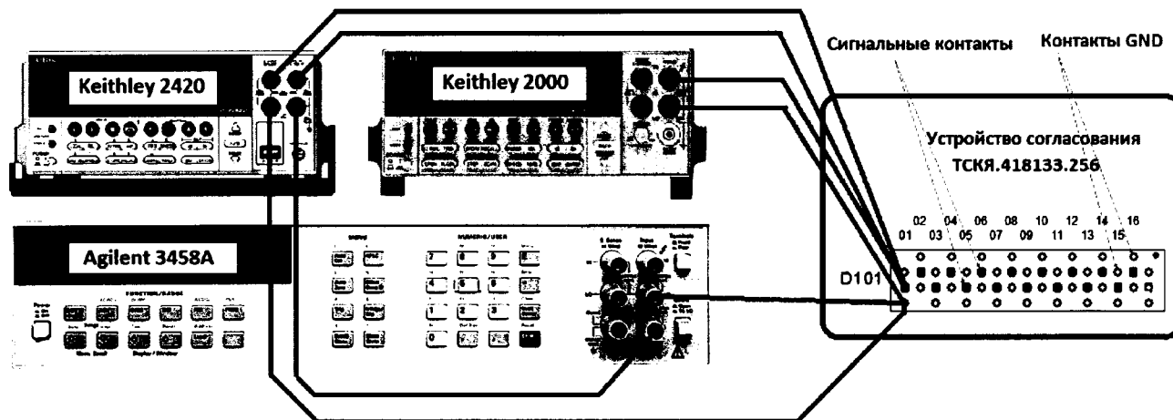
Рисунок 21 – Схема определения погрешности воспроизведения (измерения) напряжения и измерения (воспроизведения) силы тока HPPMU при подключении через плату PS1600
