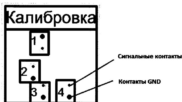
Рисунок 13 – Контакты для калибровки устройства ТСКЯ.418133.254
